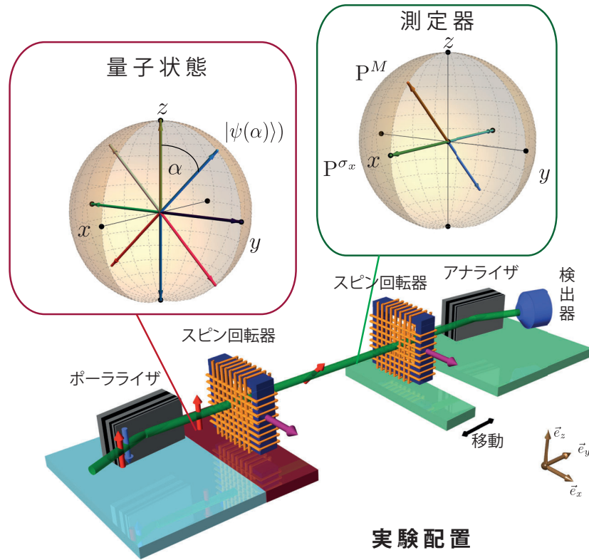
図2 実験配置図。実験用原子炉から取り出された中性子は、青の部分にあるポラライザで状態 \Psi に初期化される。次に、パラメータ掃引法を実行するために赤の部分にあるスピン回転器で初期状態をパラメータ値 t だけ変化させて \Psi(t)=U(t)\Psi に変換する。緑の部分では、3状態法に必要な操作を行った後に、アナライザでスピン測定を行う。これらの測定によって得られたデータから、状態 \Psi(t) における量子二乗平均平方根誤差の値を計算する。
